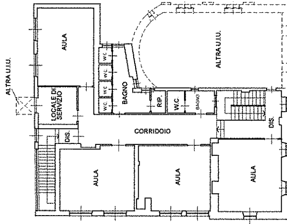
PIANTA PIANO PRIMO Hmin= 3.15 mt. Hmax= 3.60 mt.
