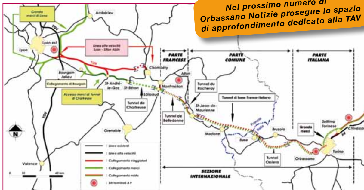
Planimetria generale della nuova linea Torino-Lione
